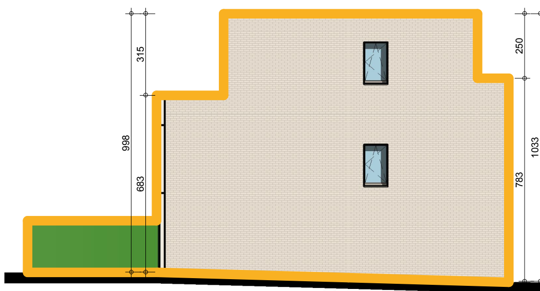
linker zijgevel
