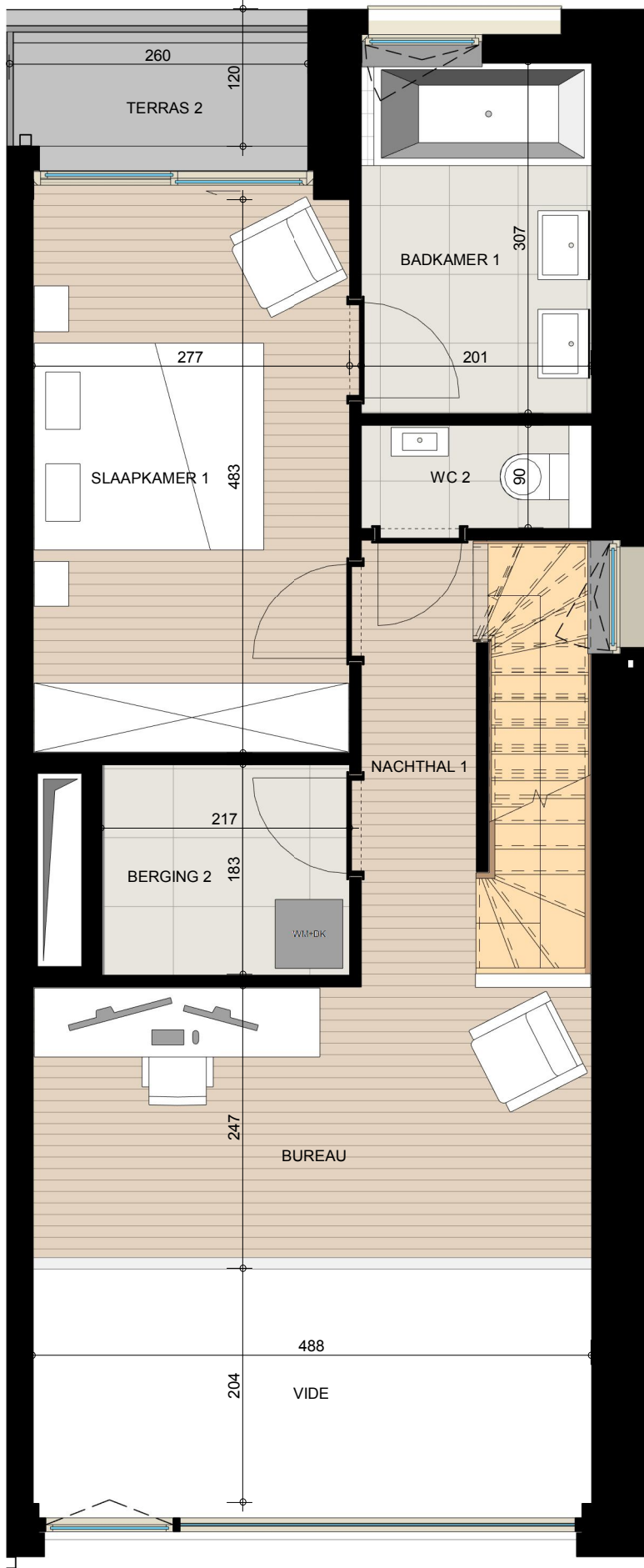
plan niv.+1
